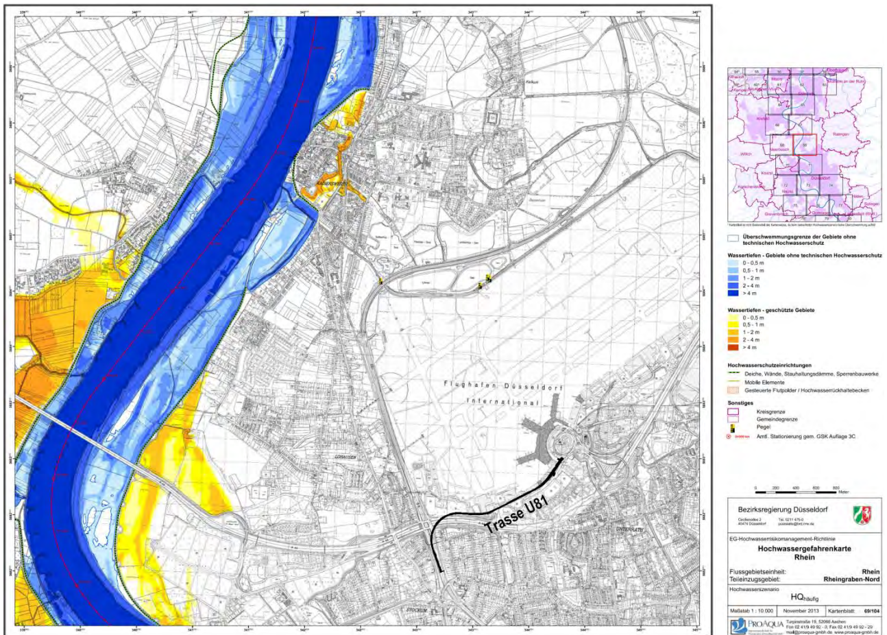
Abbildung 1: Auszug aus der Hochwassergefahrenkarte Rhein, HQhäufig [U 3]
