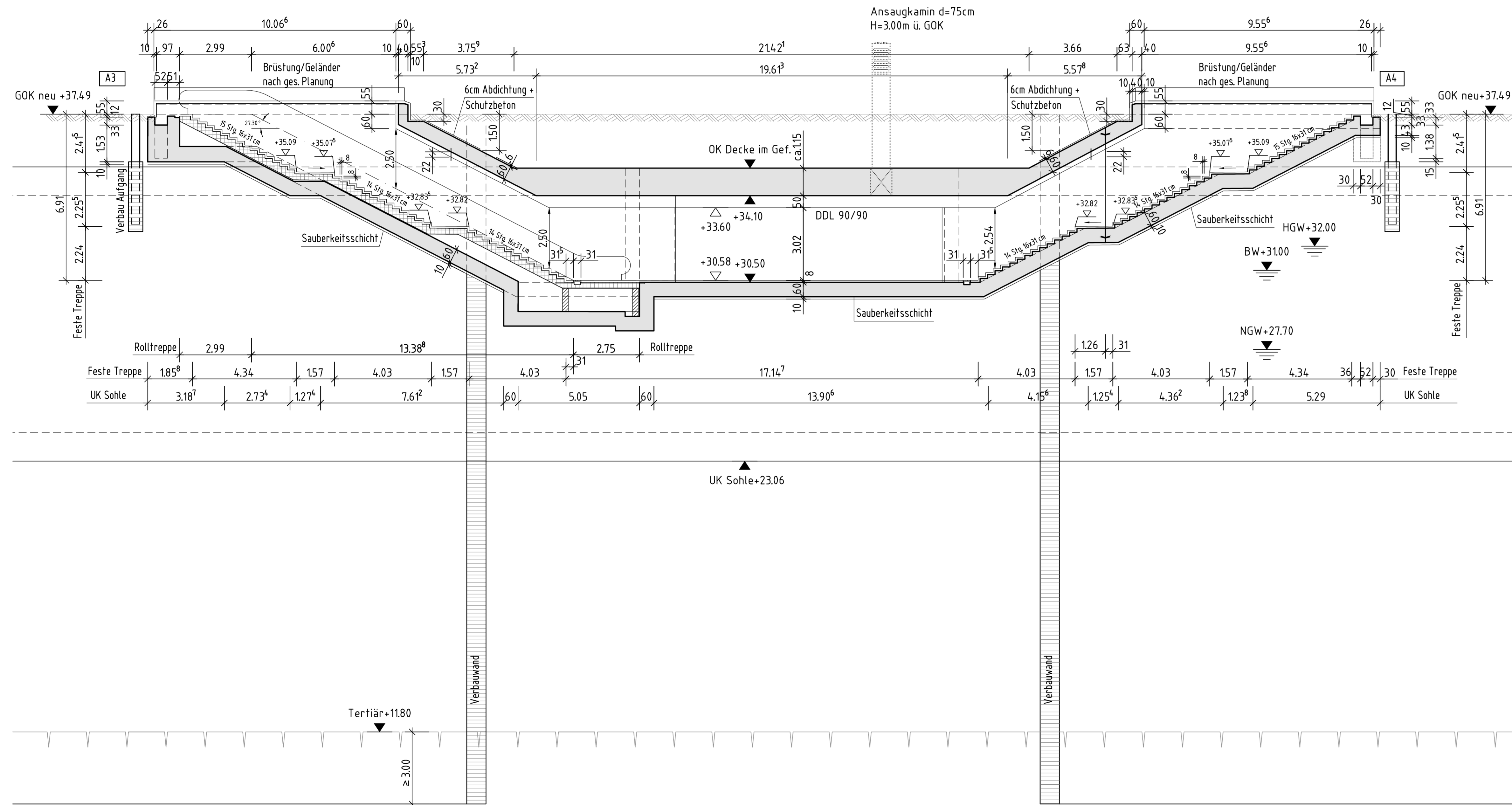
Querschnitt Q11-6, Südkopf A3 - A4 M 1:100
