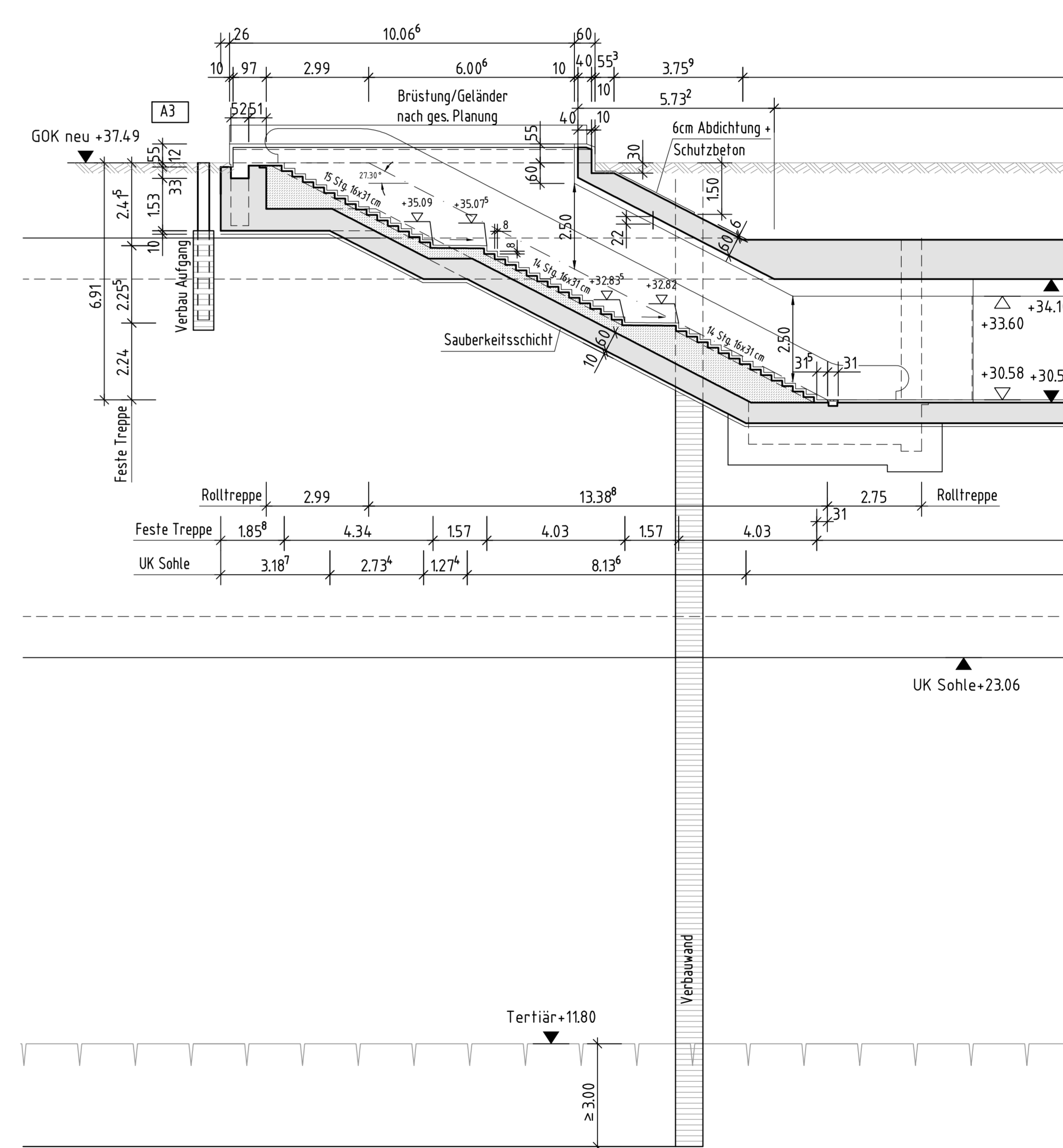
Querschnitt Q11-6.1 M 1:100
