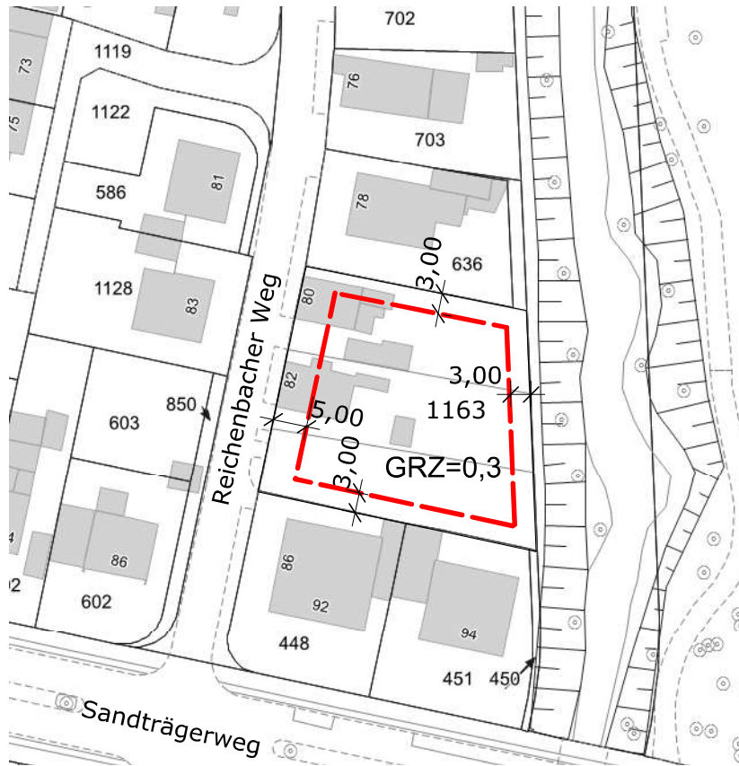
Reichenbacher Weg 80, 82 Baufenster M. 1:1.000
