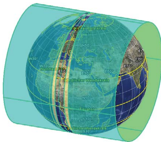
Abb. 3: Schnittzylinder der UTM-Abbildung (Zone und Schnittfläche überproportional dargestellt) Erddarstellung © 2008 Google
