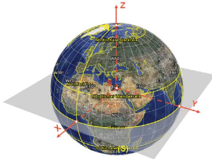
Abb. 1: Dreidimensionales kartesisches geozentrisches Koordinatensystem Erddarstellung © 2008 Google
