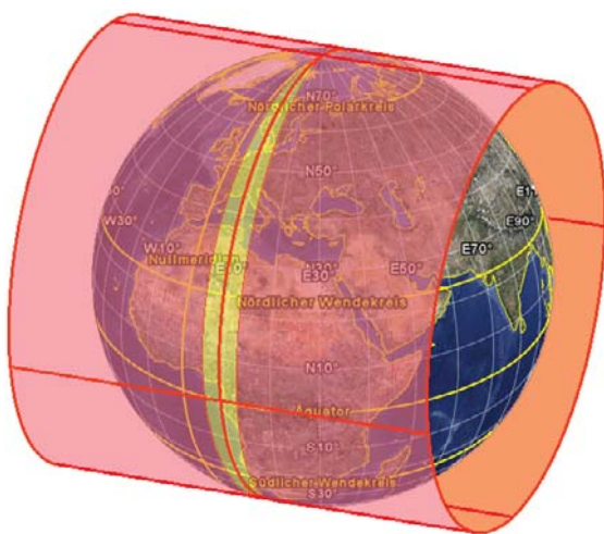
Abb. 2: Berührungszylinder der Gauß-Krüger-Abbildung (Meridianstreifen überproportional dargestellt) Erddarstellung © 2008 Google
