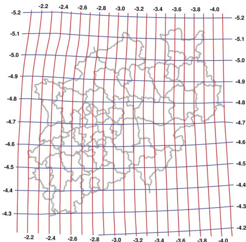
Abb. 7: Ausschnitt für Nordrhein-Westfalen aus dem Isolinienmodell der Gitterdatei des BeTA2007; Darstellung der Shiftwerte in Sekunden (Blau = \Delta B , Rot = \Delta L )
