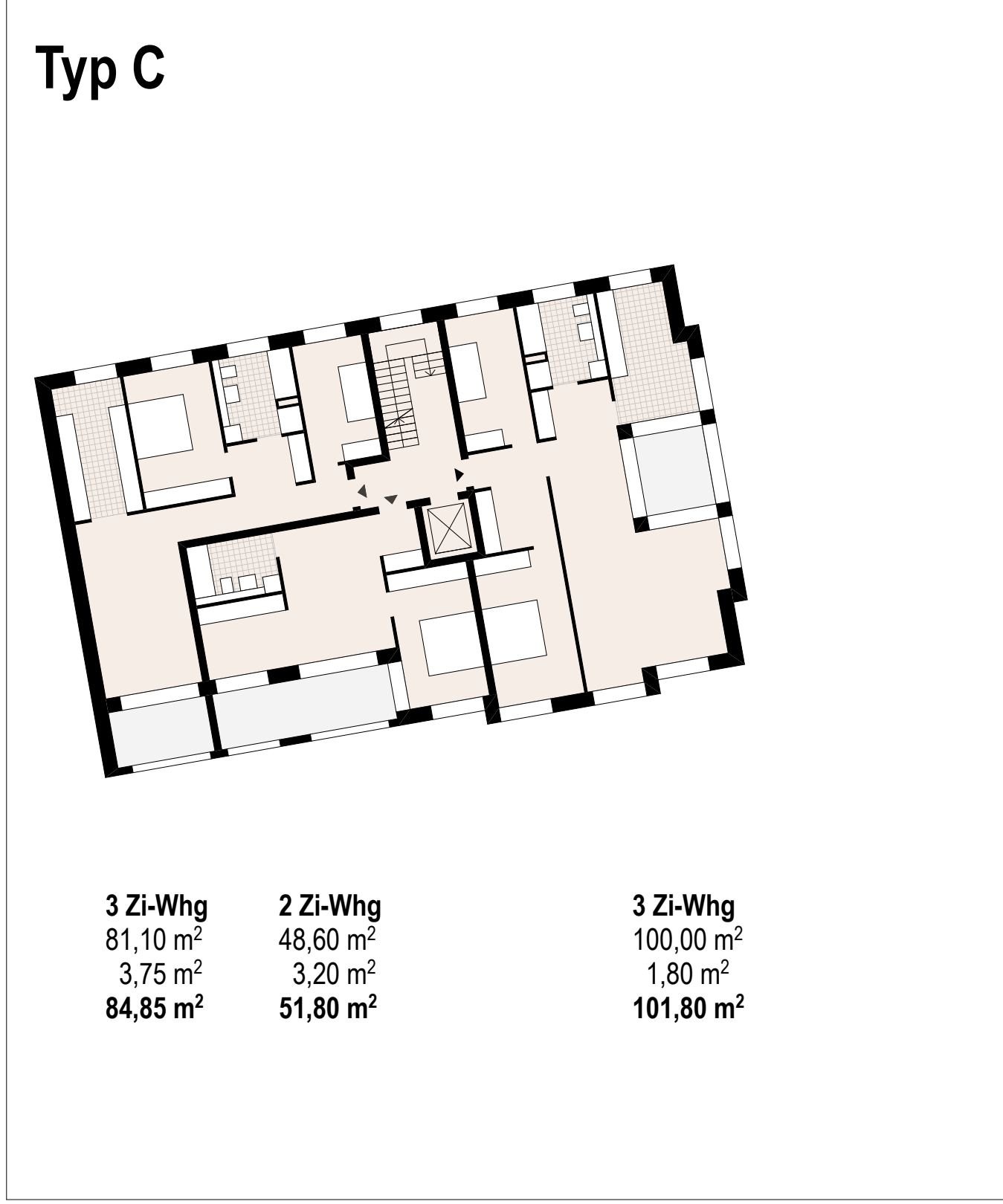
Grundriss Regelgeschoss Gebäudetypen M 1:200
