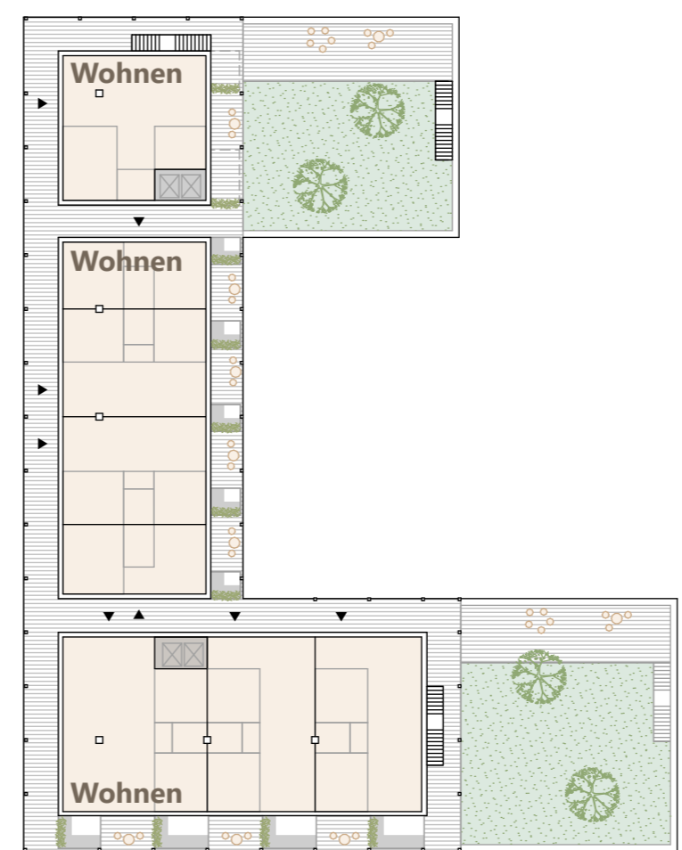
REGELGESCHOSS IN AUFSTOCKUNG M 1:500
