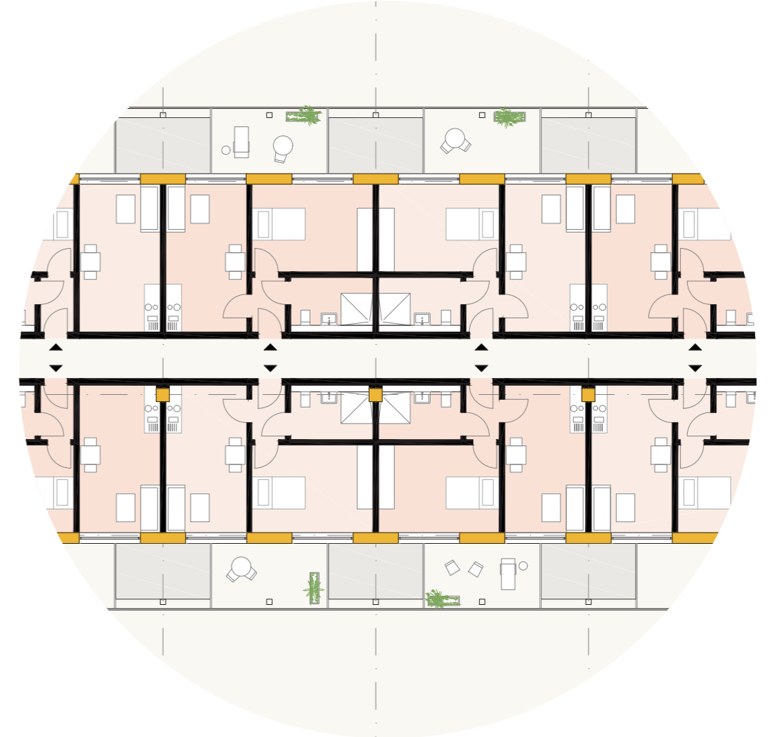
SENIORENWOHNEN M 1:200
