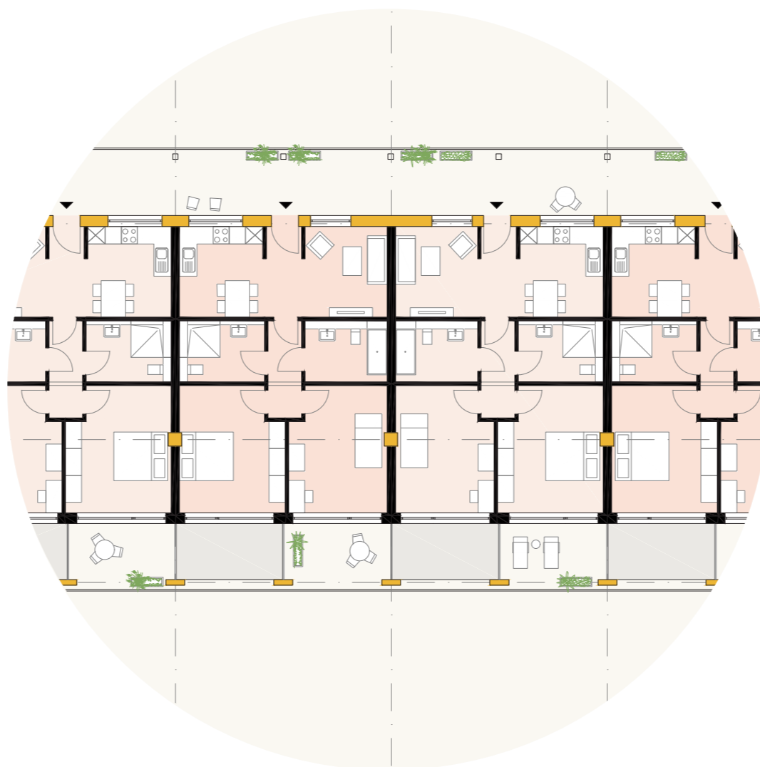
3-ZIMMER WOHNTYPOLOGIE M 1:200
