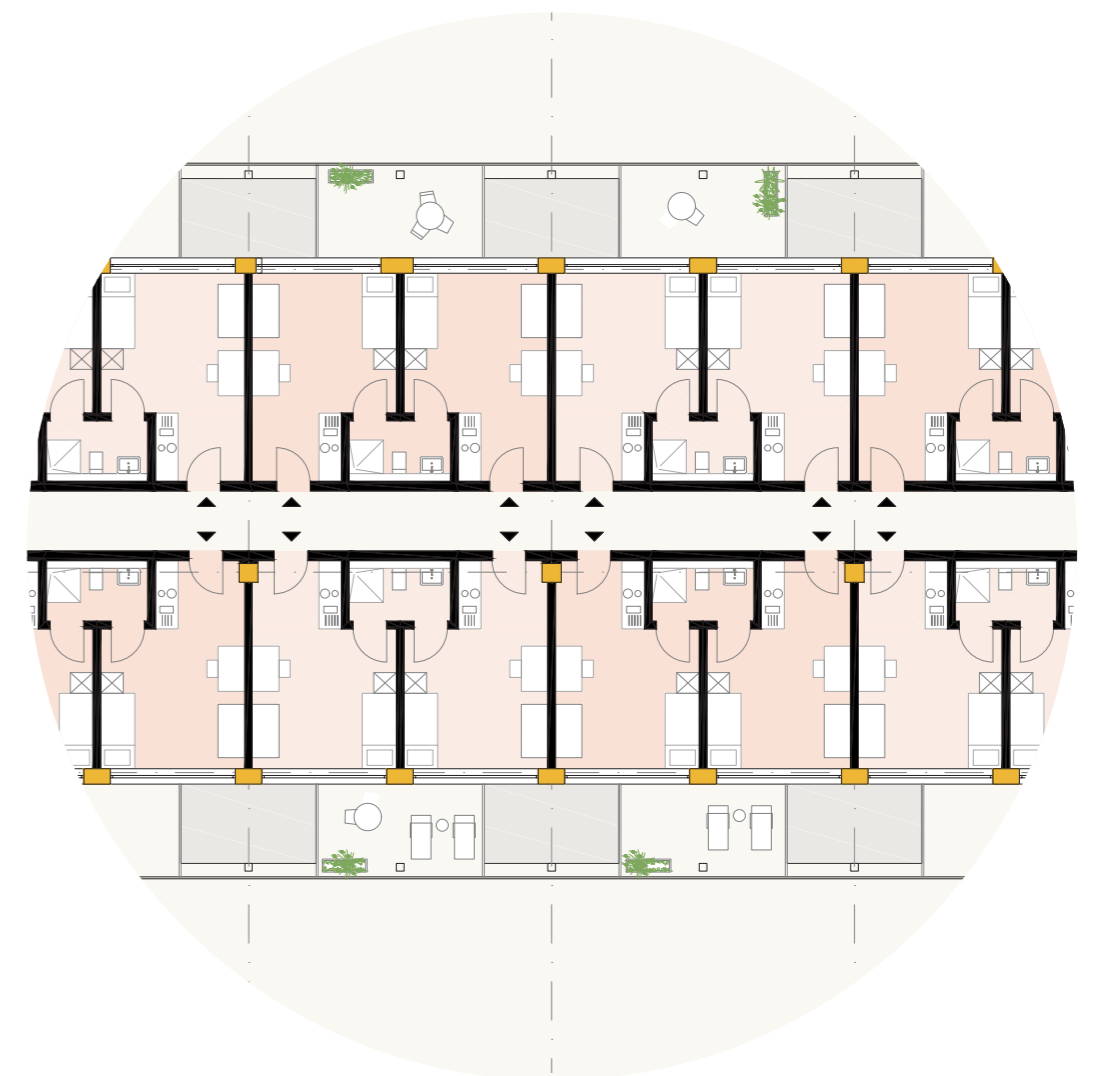
STUDENTENWOHNEN M 1:200
